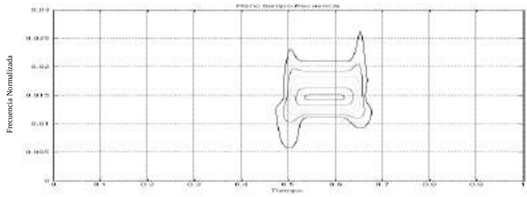
a. Transformada S corriente i_A(t)
