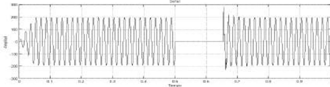
b. Tensión de línea v_{AN}(t)
