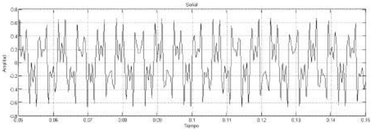
Figura 10. Señal de corriente medida en el neutro.
