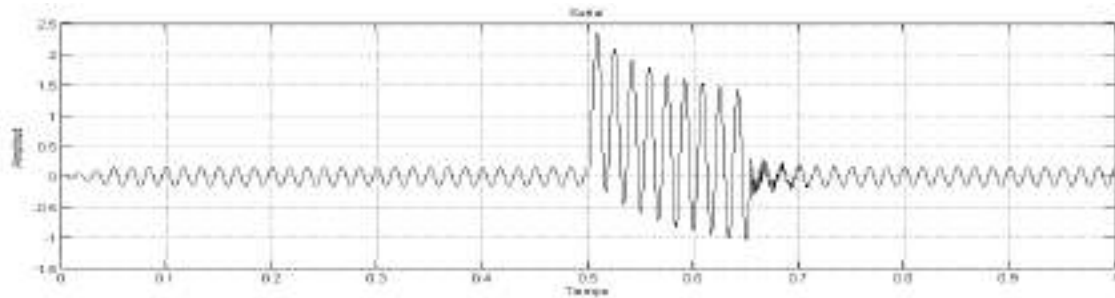
a. Corriente i_A(t)
