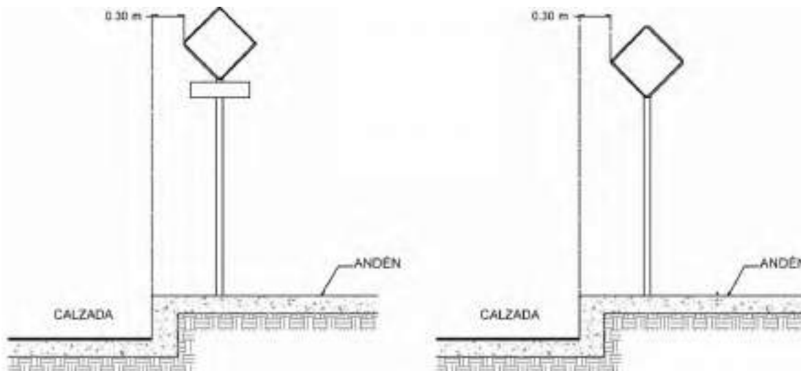
Figura 29 Ubicación lateral de una señal sobre andén
