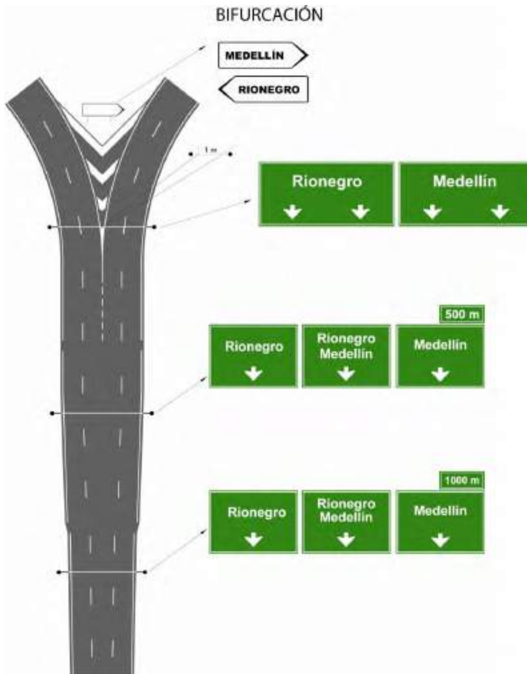
Figura 133. Bifurcación en autopista
