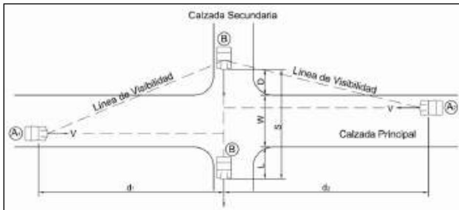
Figura 124. Distancia de visibilidad en intersecciones.
