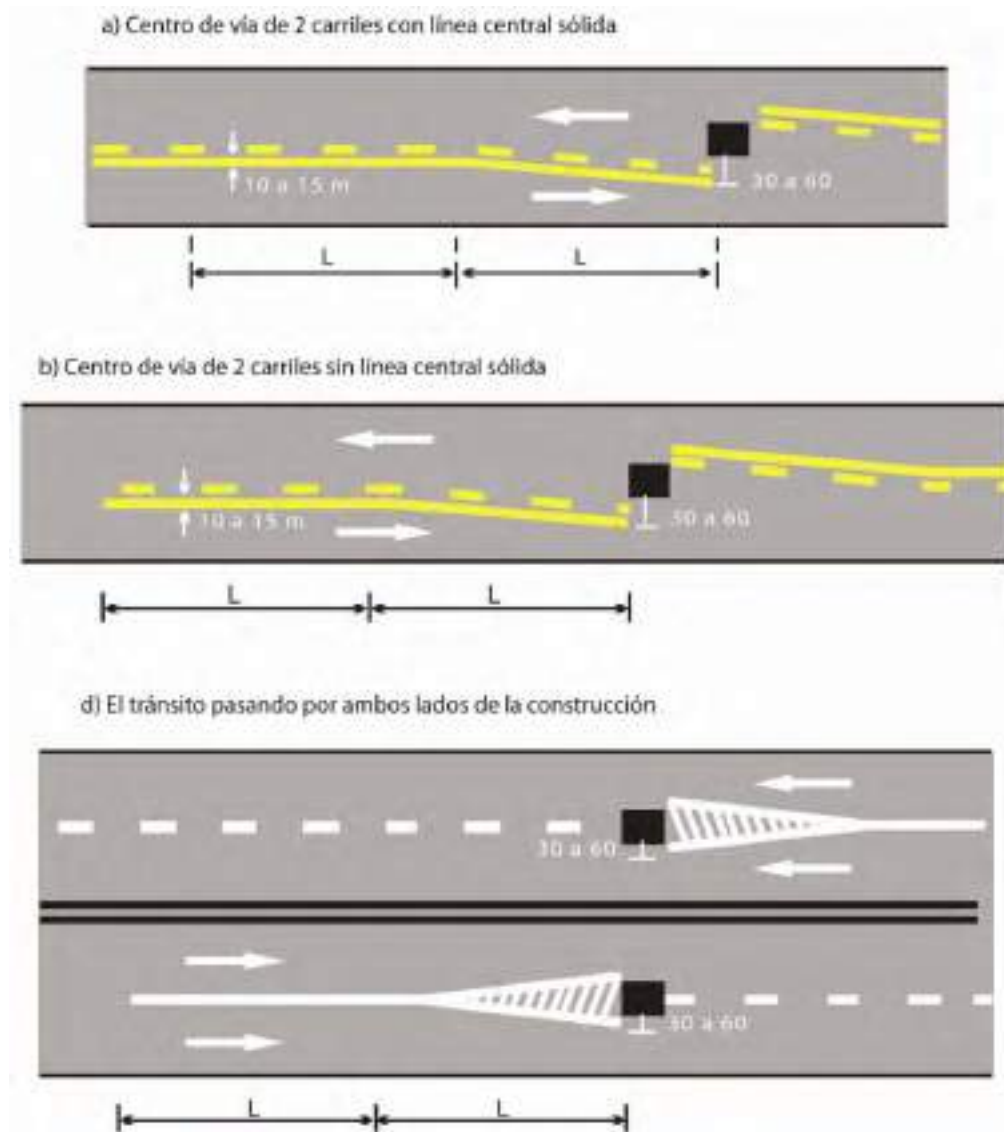
Figura 161. Demarcación de aproximación a obstrucciones
