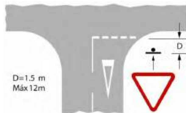
Figura 91. Señal de Ceda el paso en intersección
