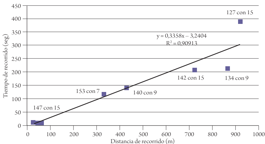
Figura 5. Distancia frente a tiempo de recorrido: giro a la izquierda
