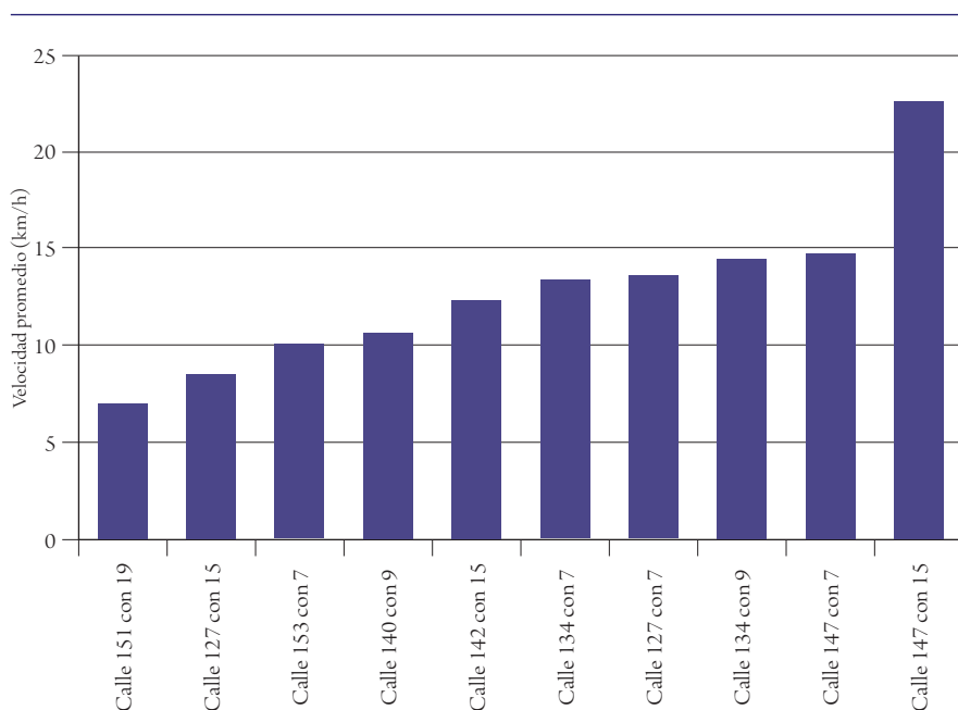
Figura 6. Velocidad promedio: giro a la izquierda
