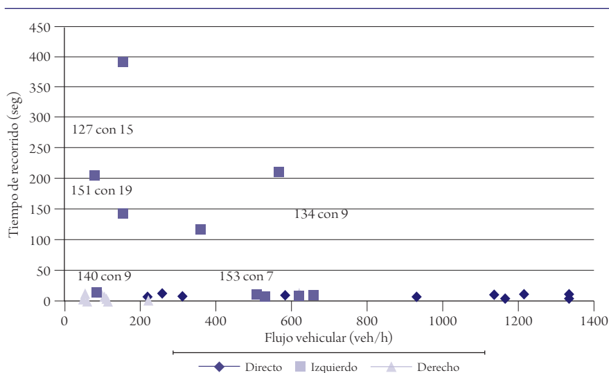
Figura 4. Flujo vehicular frente a tiempo de recorrido
