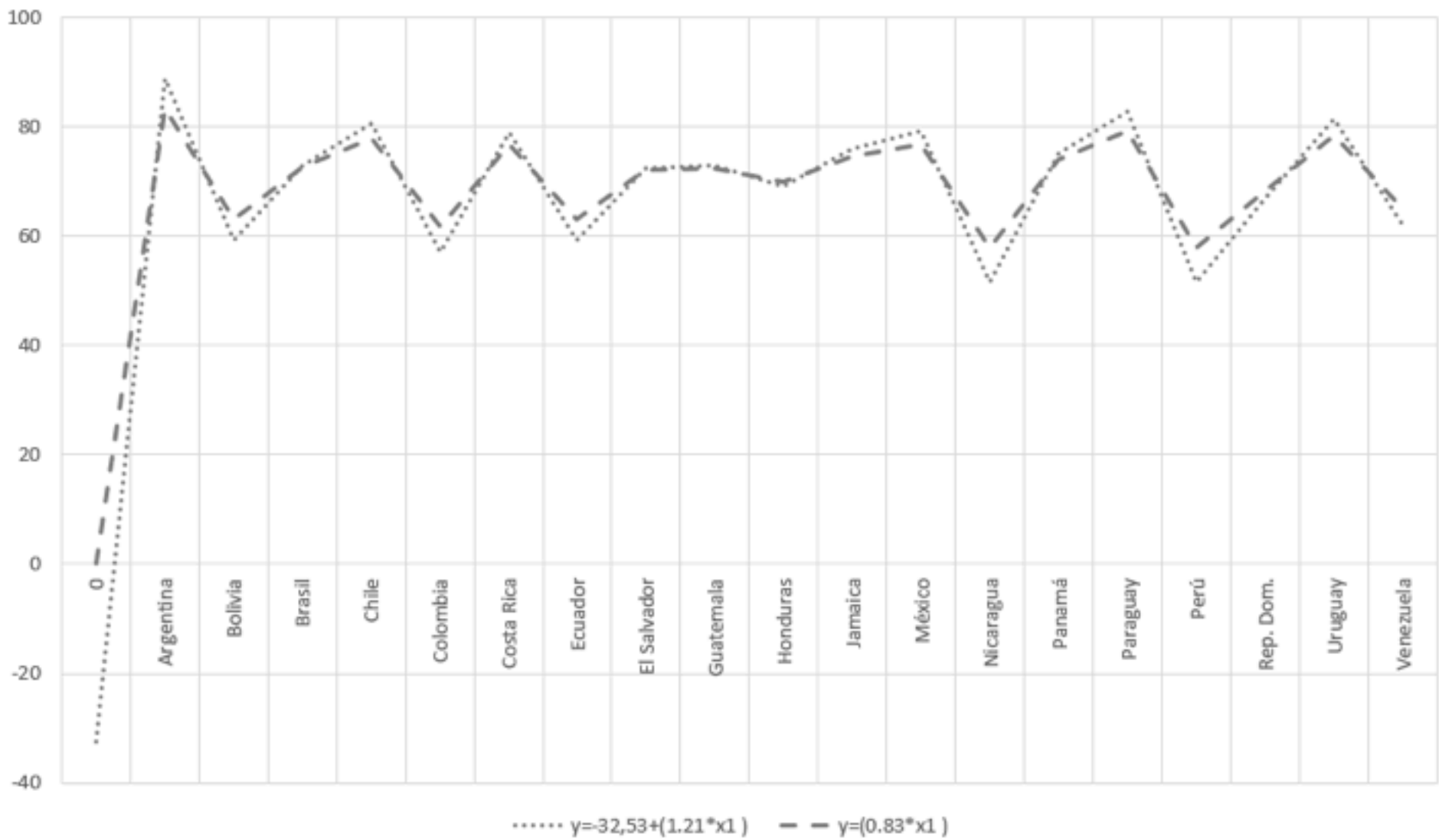
Figura 3 Modelos que emplean la cobertura del servicio de agua potable en zonas rurales como única variable explicativa a la cobertura del servicio de saneamiento mejorado en zonas rurales, ecuaciones 4 y 5. Cifras 2015.
