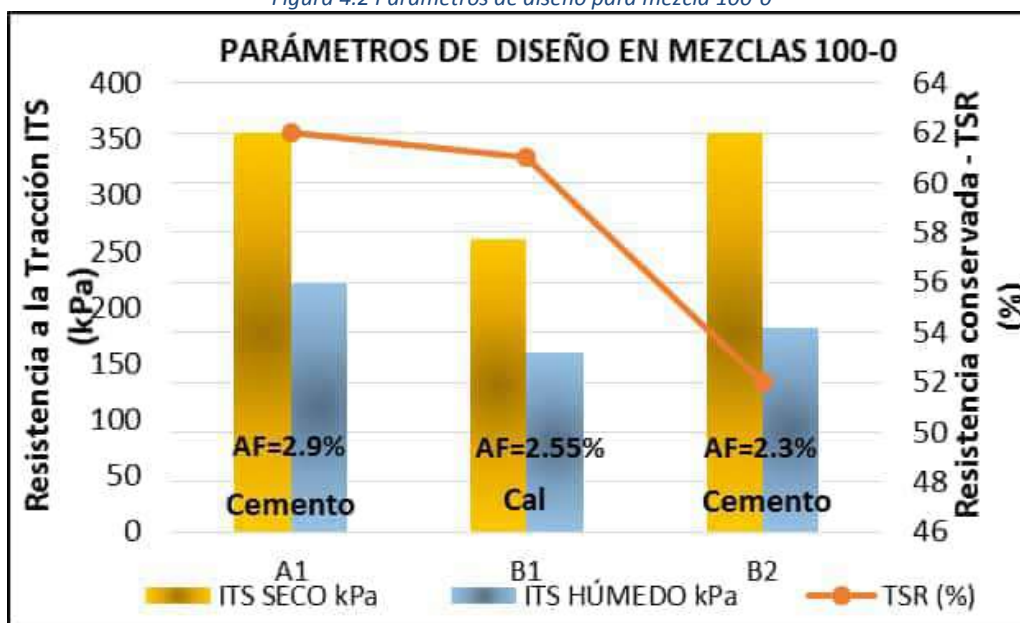
Figura 4.2 Parámetros de diseño para mezcla 100-0
