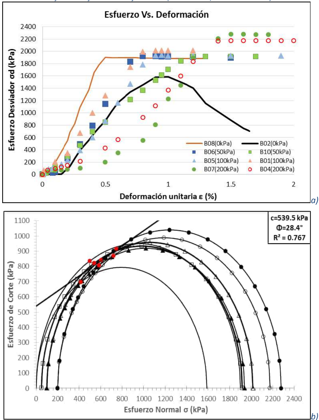
Figura 5.2.2 a) Curvas esfuerzo de formación b) Envolvente de falla Mohr – Coulomb para la mezcla 85-15 AF-B1 con diferentes esfuerzos de confinamiento (0 kPa, 50 kPa, 100 kPa Y 200 kPa)
