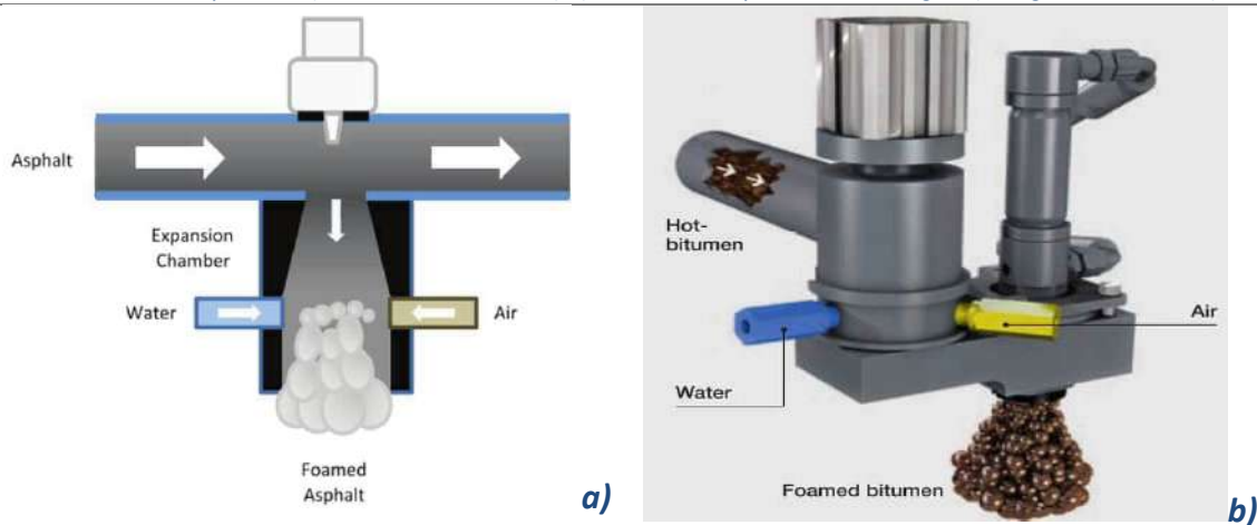
Figura 2.1 Esquema de Cámara de Expansión de Espuma y Sistema de Espumado. a) Ilustración de la vista interna de la Cámara de Expansión. (Newcomb et al., 2015) b) Sistema de Espumado de Wirtgen. (Wirtgen GmbH, 2009)
