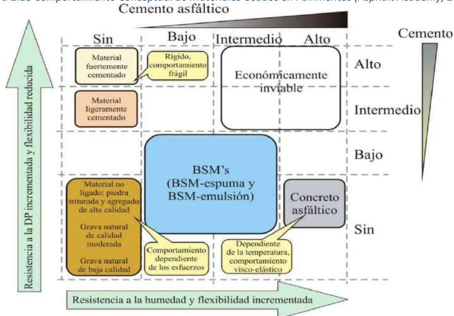
Figura 2.18 Comportamiento Conceptual de Materiales Usados en Pavimentos (Asphalt Academy, 2009b)
