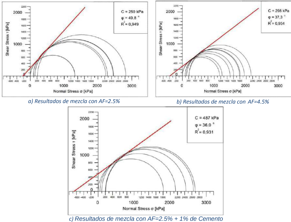
Figura 2.25 Resultados de ensayos realizados por Cizkova
