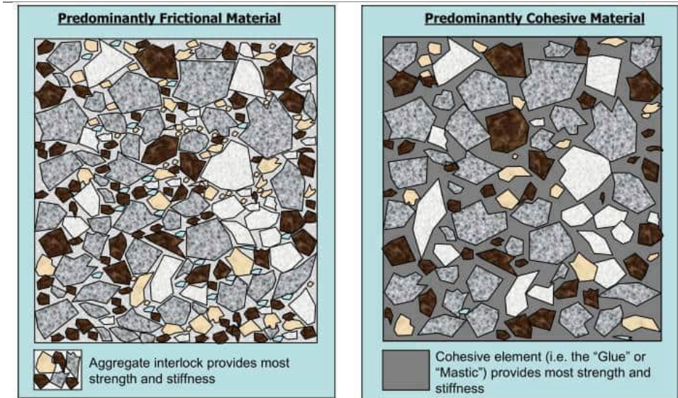
Figura 2.23 Esquema representativo de material Predominantemente Friccional (Izq.) y material Predominantemente Cohesivo. (Der.) (Jooste et al., 2007)
