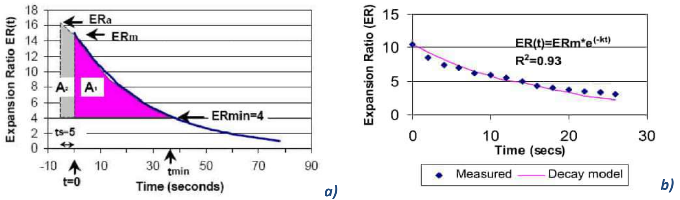
Figura 2.7 a). Área Bajo curva de decaimiento de la espuma. b). Modelo exponencial y datos medidos. (K.J. Jenkins, 1999)
