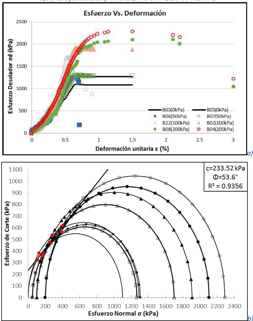
Figura 5.2.2 a) curvas esfuerzo de formación (b) Envolvente de falla Mohr – Coulomb para la mezcla 100-0 AF-B2 con diferentes esfuerzos de confinamiento (0 kPa, 50 kPa, 100 kPa Y 200 kPa)
