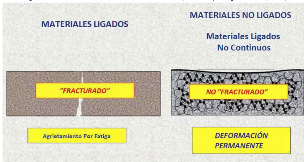
Figura 2.19 Condiciones de Falla en el Pavimento. Adaptado de: (Collings & Jenkins, 2012)
