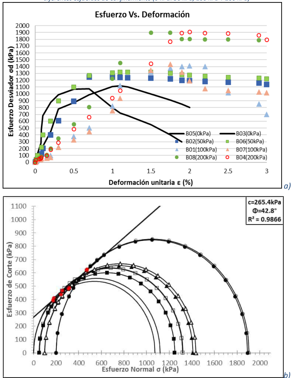
Figura 5.2.2 a) Curvas esfuerzo de formación (b) Envolvente de falla Mohr – Coulomb para la mezcla 70-30 AF-B2 con diferentes esfuerzos de confinamiento (0 kPa, 50 kPa, 100 kPa Y 200 kPa)
