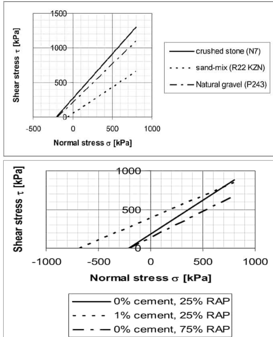
Figura 2.30. Envolventes de resistencia para diferentes materiales. (Ebels & Jenkins, 2007b)
