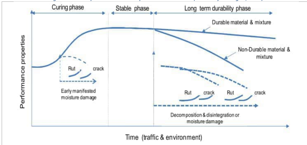
Figura 2.35 Comportamiento Conceptual de los BSM-AF. (Mathaniya Twagira, 2010)
