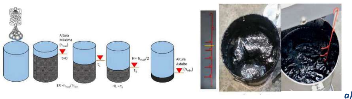
Figura 2.12 Métodos de medición Invasiva de Propiedades a) Método de la varilla Graduada. b) Método AFCT. (Ozturk, 2013). c) Curvas de Decaimiento Obtenidas Mediante Técnica AFCT. (Campagnoli et al., 2016)
