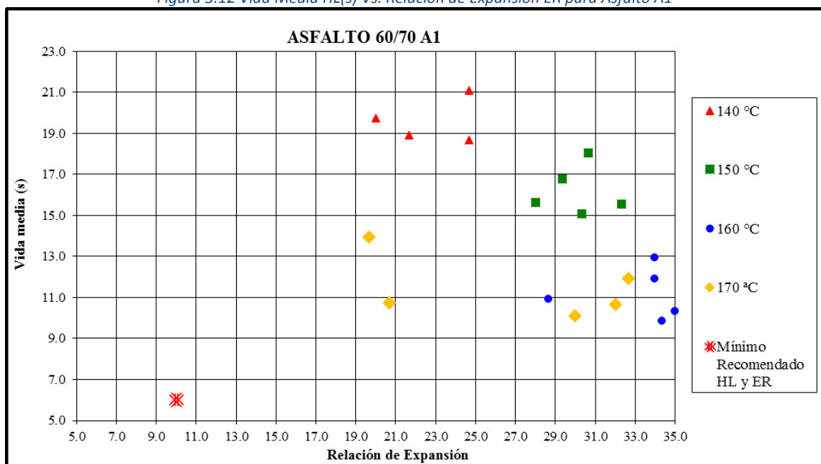
Figura 3.12 Vida Media HL(s) Vs. Relación de Expansión ER para Asfalto A1
