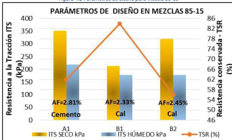
Figura 4.2 Parámetros de diseño para mezcla 85-15
