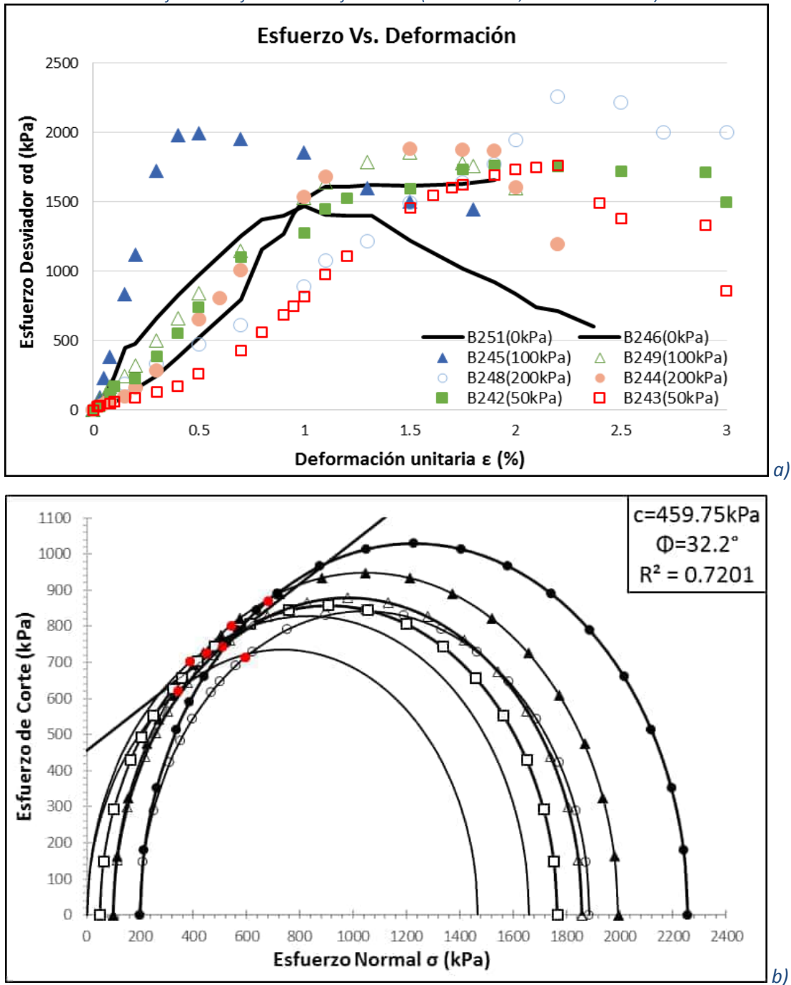
Figura 5.2.2 a) Curvas esfuerzo deformación b) Envolvente de falla Mohr – Coulomb para la mezcla 100-0 AF-B1 con diferentes esfuerzos de confinamiento (0 kPa, 50 kPa, 100 kPa Y 200 kPa)
