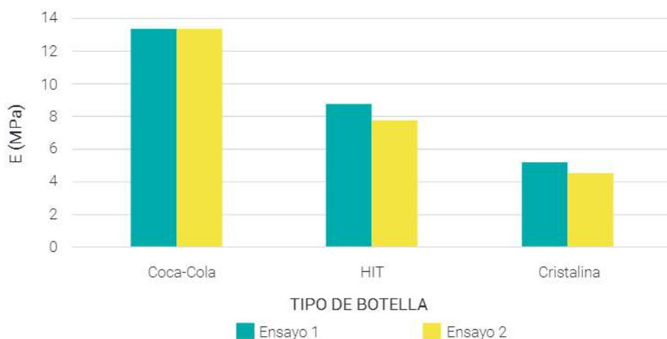
Figura 9. Comparación módulo de elasticidad de cada tipo de botella. Fuente: elaboración propia.
