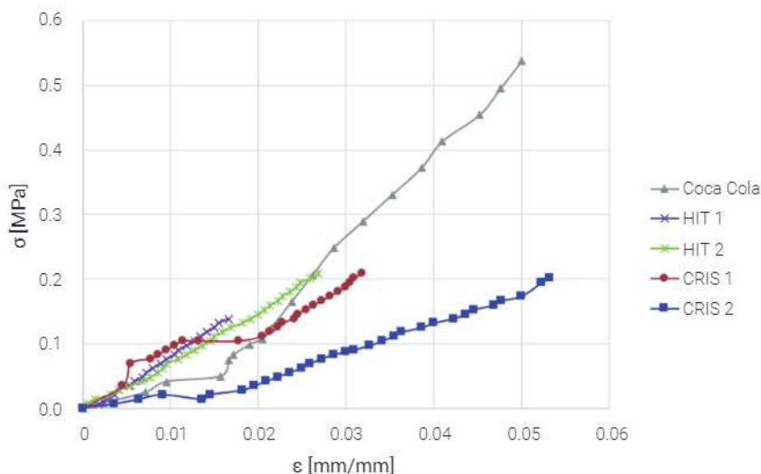
Figura 8. Curva esfuerzo vs. deformación unitaria para el ensayo a carga axial. Fuente: elaboración propia.
