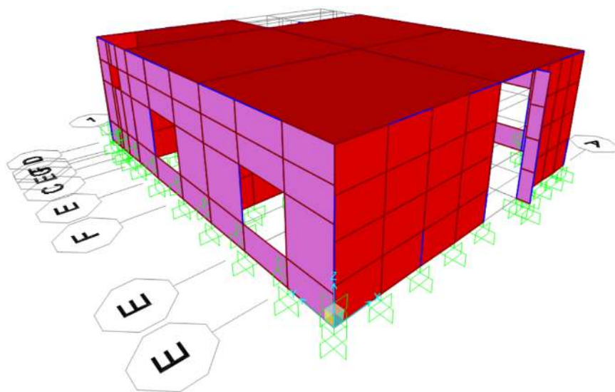
Figura 14. Modelo en elementos finitos (EF).
