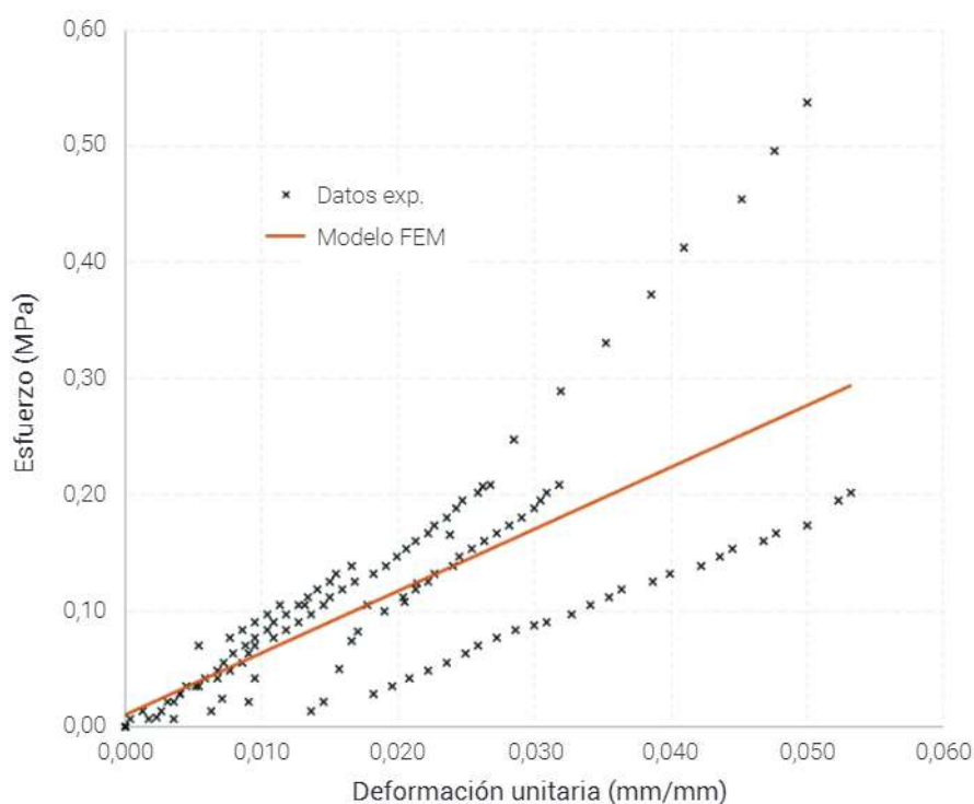
Figura 12. Comparación de las curvas esfuerzo-deformación experimental vs. modelo. Fuente: elaboración propia.
