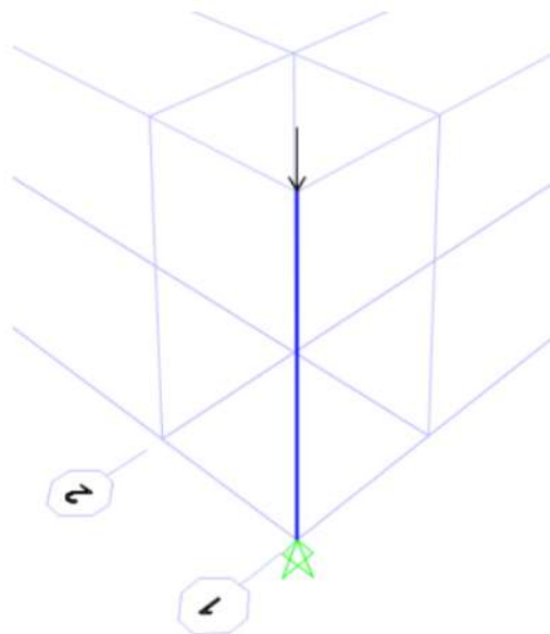
Figura 11. Modelo simplificado en elementos finitos del ensayo de laboratorio. Fuente: elaboración propia.
