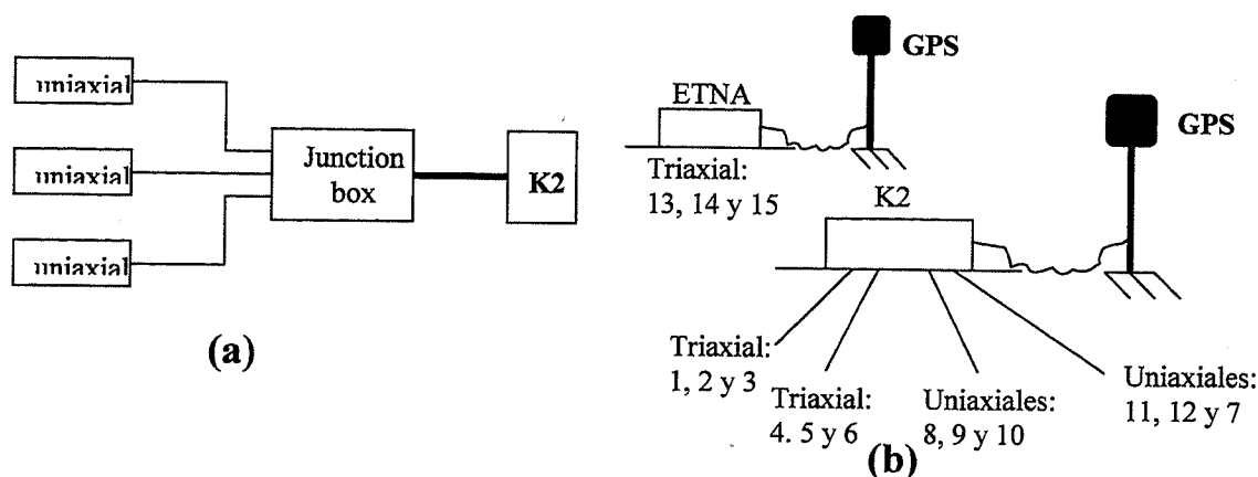
Figura 20: Esquema de interconexión de la instrumentación en la represa La Plata: (a) Conexión de los sensores uniaxiales; (b) Conexión de todo el sistema.
