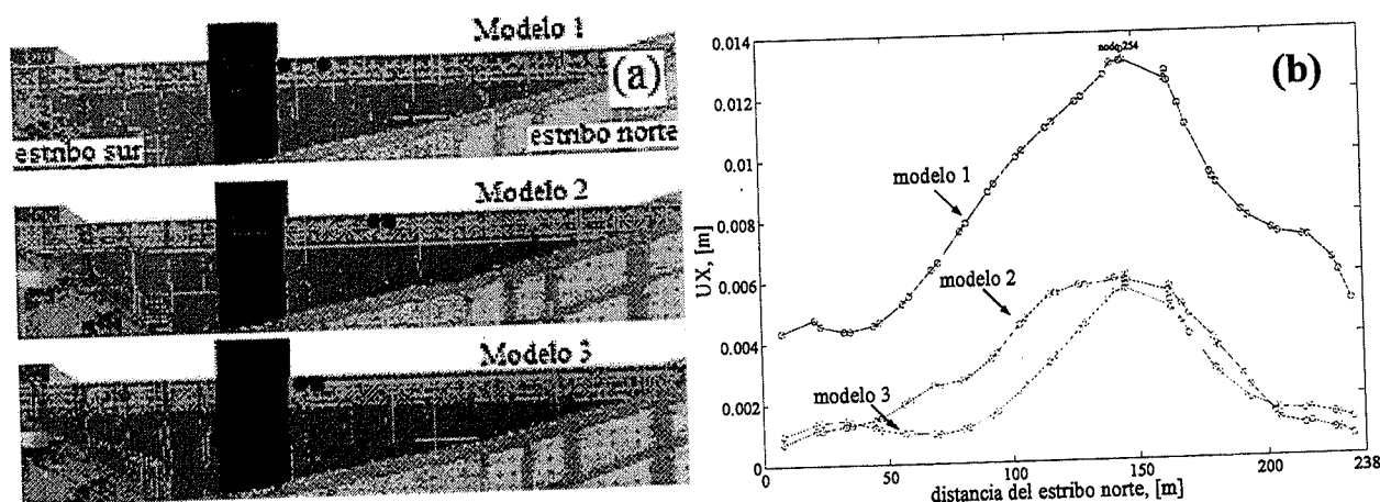
Figura 11: Desplazamientos máximos en la dirección X ante el evento máximo creíble: (a) Vista hacia aguas abajo; (b) Envolvente de desplazamientos a nivel de la cresta.
