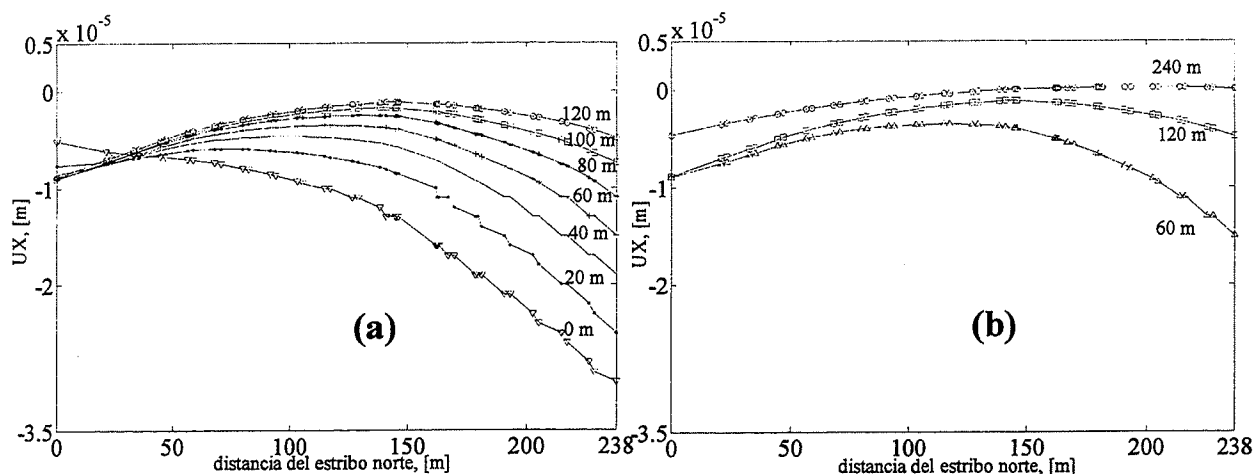
Figura 9: Variación del primer modo de vibración de la dirección longitudinal al río para un eje a lo largo de la cresta, usando un modelo de roca con masa: (a) Hasta 120 de malla de suelo a cada lado; (b) Hasta 240 m de malla.
