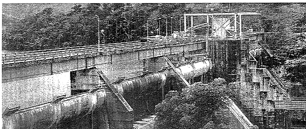
Figura 17: Instalación de los acelerómetros usando el carro con brazo mecánico.
