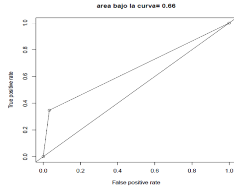
Figura. 5. Curva ROC y área bajo la curva para RF
