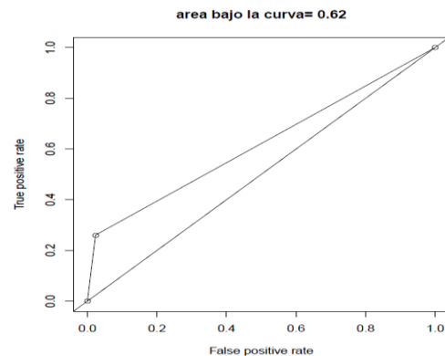
Figura. 7. Curva ROC y área bajo la curva para SVR
