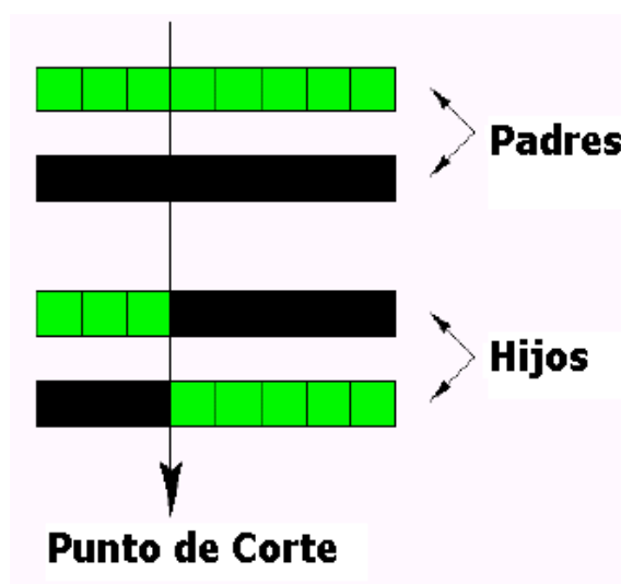
Figura II.9. Cruzamiento de un punto (one-point crossover)
