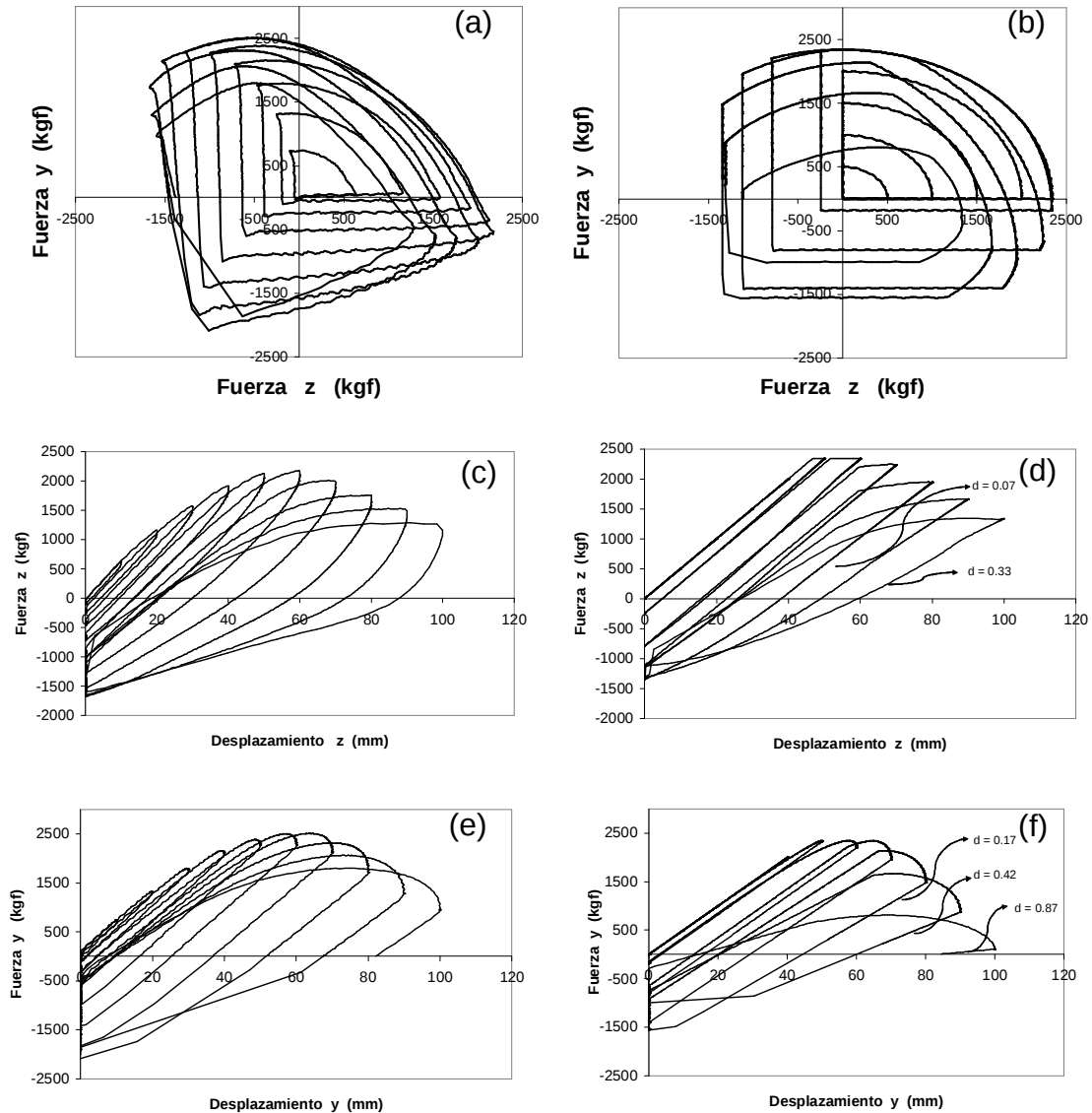
Figura 19. Resultados experimentales y de la simulación del ensayo VPTC-CC a) Fuerza z – Fuerza y experimental. b) Simulación numérica. c) Fuerza – Desplazamiento experimental en la dirección z . d) Simulación numérica. e) Fuerza – desplazamiento experimental en la dirección y . f) Simulación numérica
