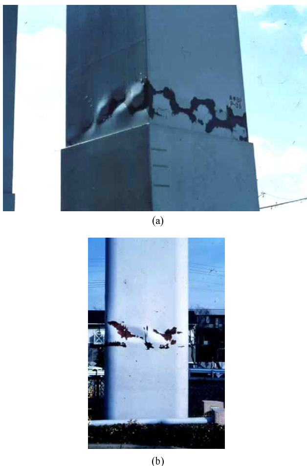
Figura 1. Columnas afectadas por pandeo local durante el terremoto de Kobe
