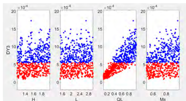
Drift Y – level 3
