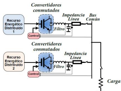
Figura 21. Dos unidades formadoras conectadas en paralelo a un bus común con la carga.
