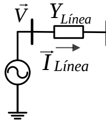
Figura 7. Modelo de unidad formadora.
