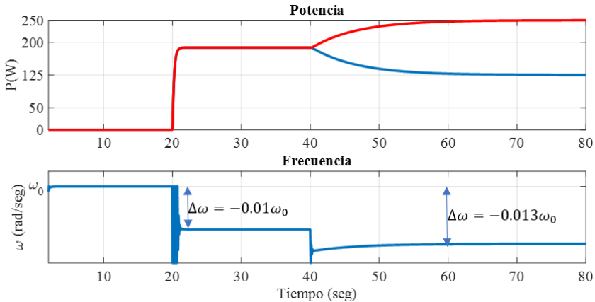
Figura 24. Respuesta en el tiempo para una microrred AC con dos unidades formadoras.
