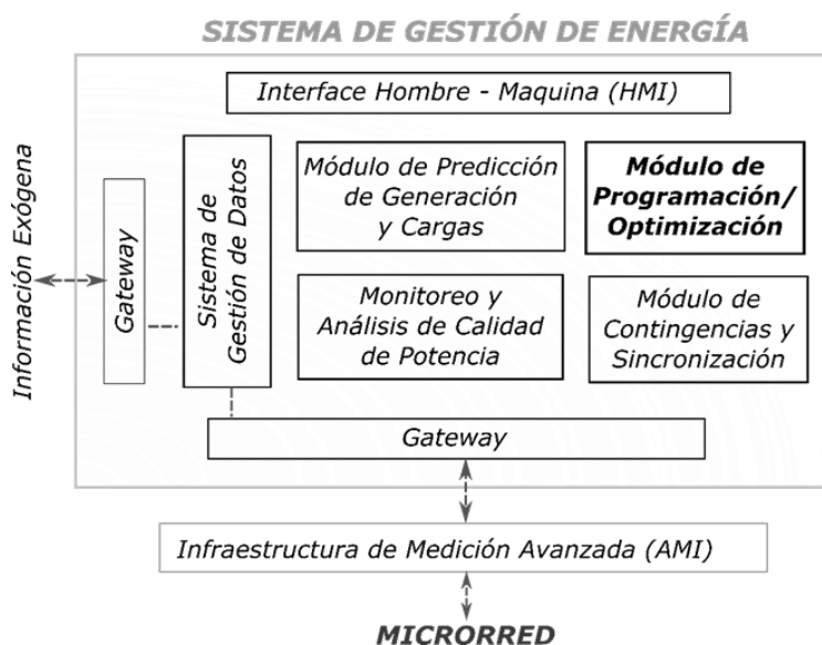
Figura 34. Ejemplo de estructura modular de un MGEMS.
