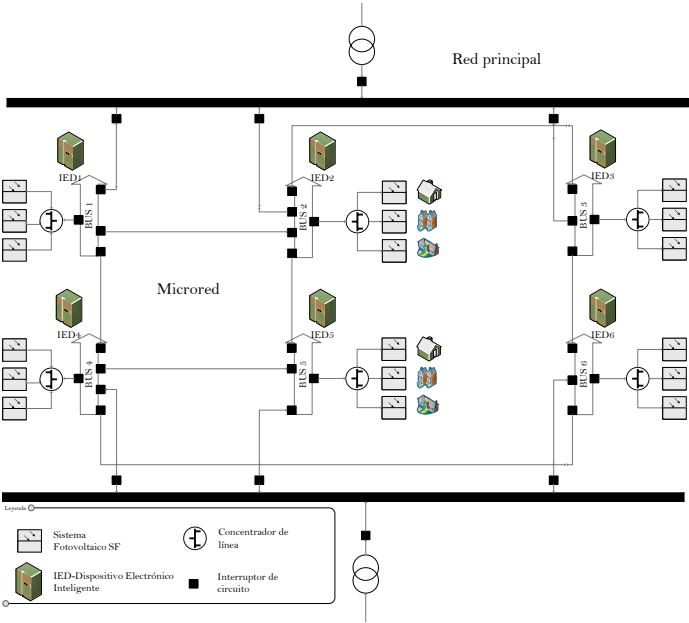
Figura 60. Esquema de coordinación por sistema de comunicación con IEDs. Ajustado de [85].
